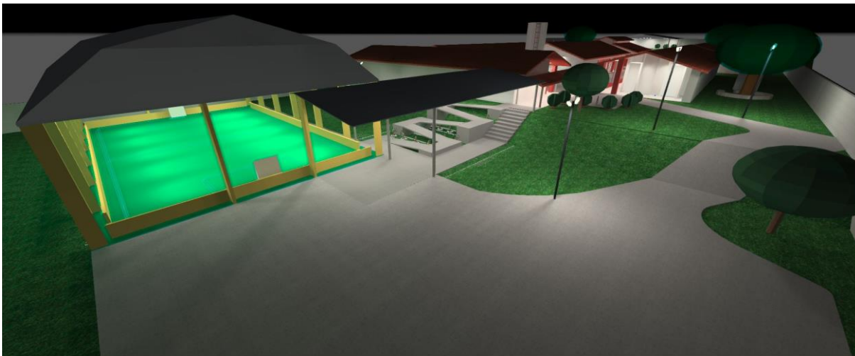
Figura 27 - Resultado da Simulação no Dialux (Cores Reais) – Estacionamento
